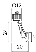
Auto Grip Lock 1,2 - 1,8 mm / 15-40 kg
