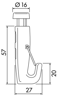
Auto Grip Lock 2,5 mm 70 kg
