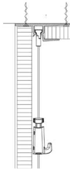
Shadowline Drywall
